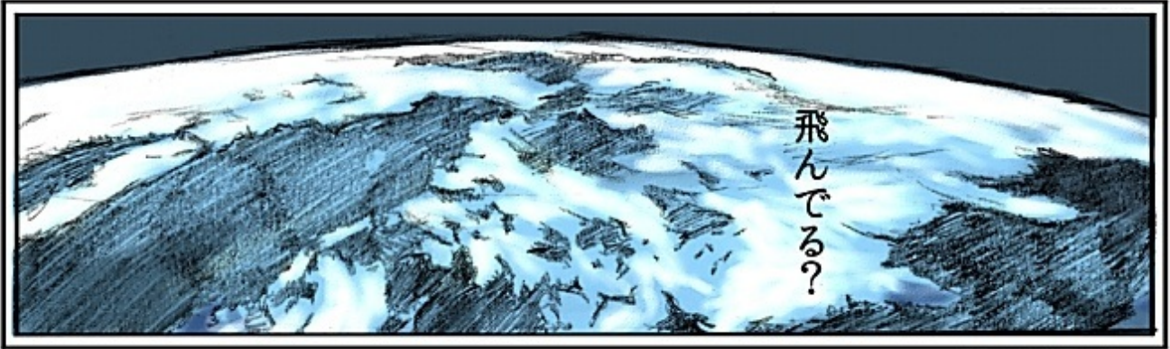
Planet Earth
